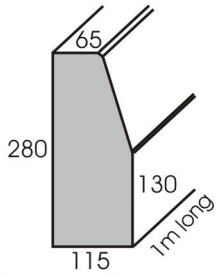
Modcon Kerbing Type 012
