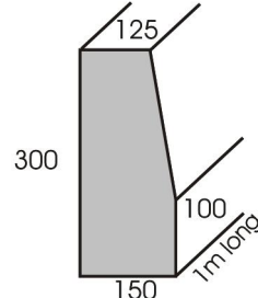
Modcon Kerbing Type 007
