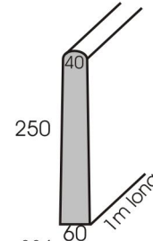
Modcon Kerbing Type 004
