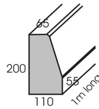
Modcon Kerbing Type 011
