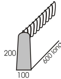
Modcon Kerbing Type 005
