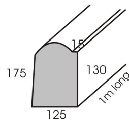
Modcon Kerbing Type 009
