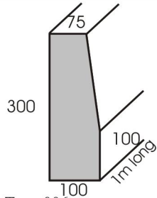
Modcon Kerbing Type 006
