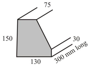
Modcon Kerbing Type 0020A
