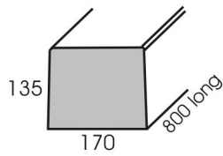
Modcon Kerbing Type 001
