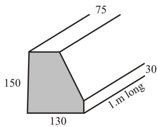
Modcon Kerbing Type 0020
