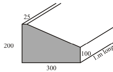
Modcon Kerbing Type 0013
