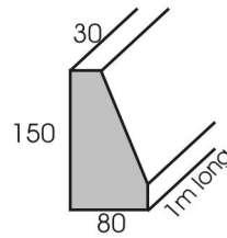
Modcon Kerbing Type 002
